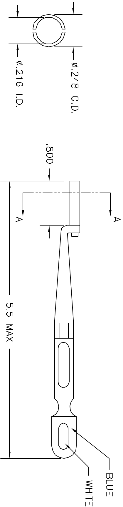
VIEW A-A
